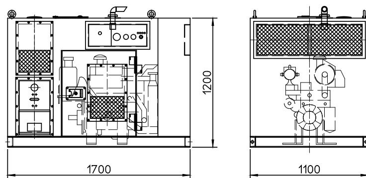
図 1-12 エンジン式油圧ユニットの外形図
