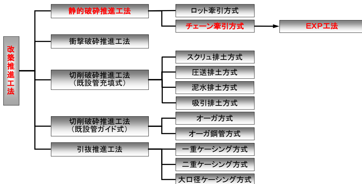
図 1-3 改築推進工法における EXP 工法の位置付け
