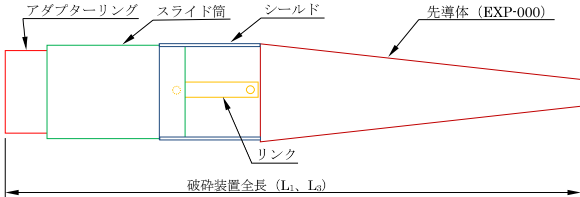
図 3-2 破砕装置図
