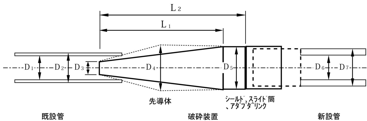
図 1-6 既設管、新設管、先導体の各部寸法
