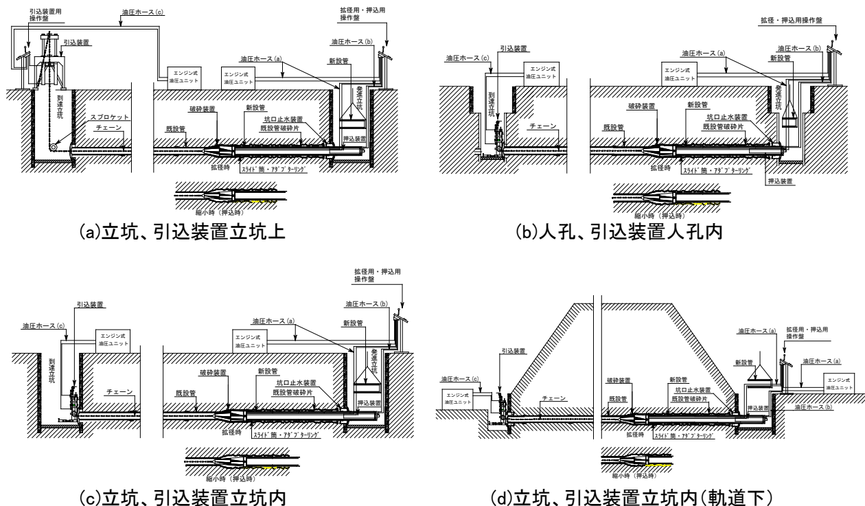
図 1-5 EXP 工法の概要図
